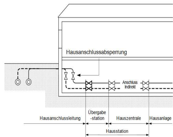
Abb. 1: Hausanschlussleitung und Hausstation nach AGFW FW 515
